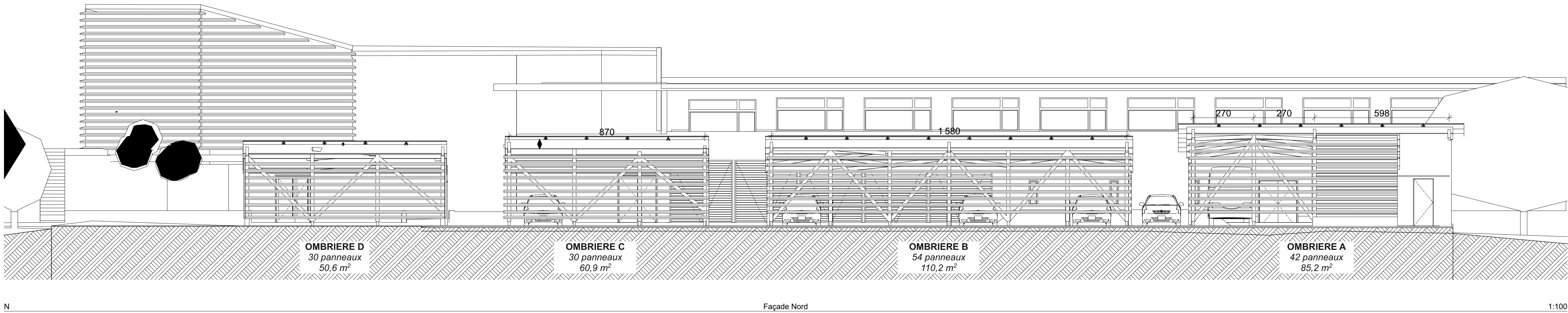
N Façade Nord 1:100
