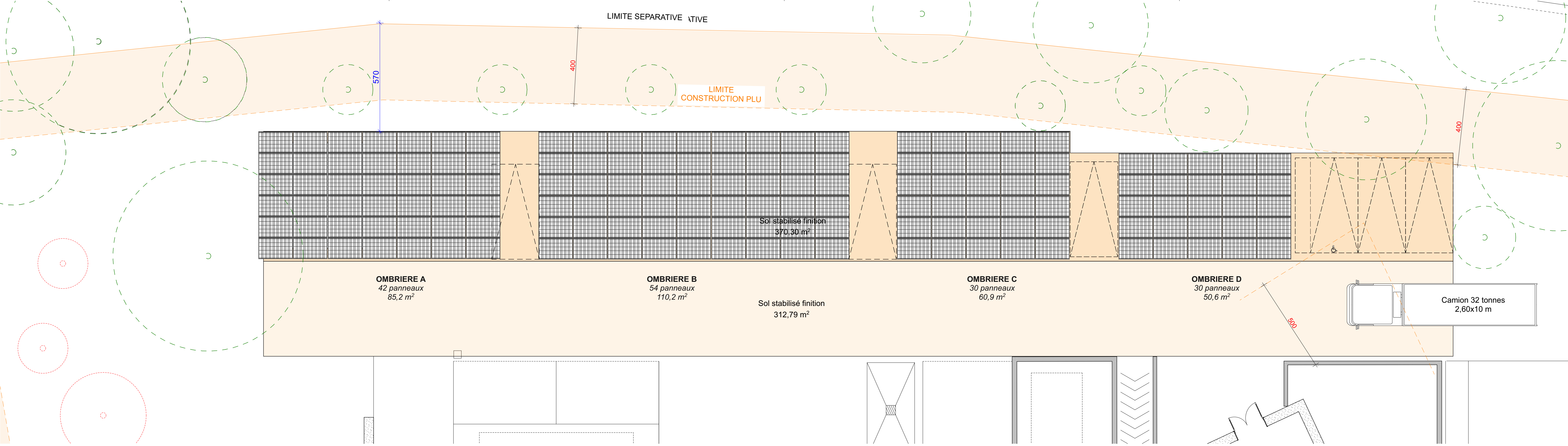
-1. Plan Toitures 1/50 1:100
